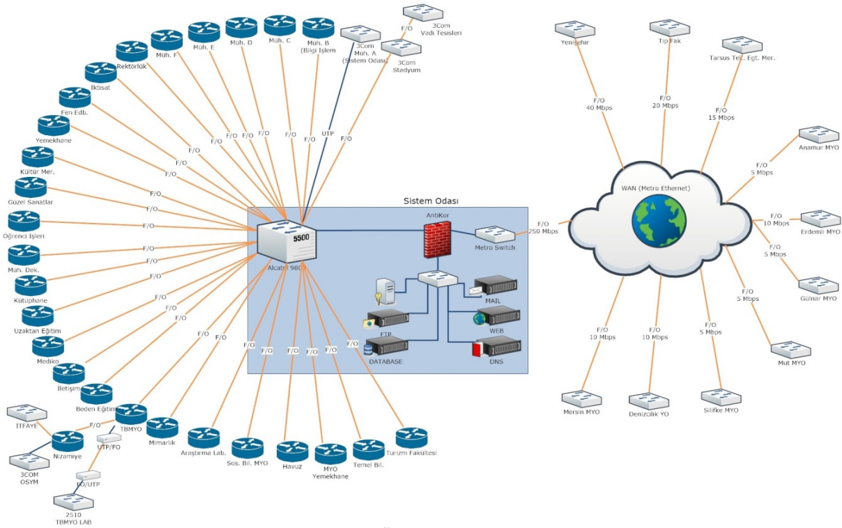
Şekil 3. Mersin Üniversitesi Ağ Topolojisi.
