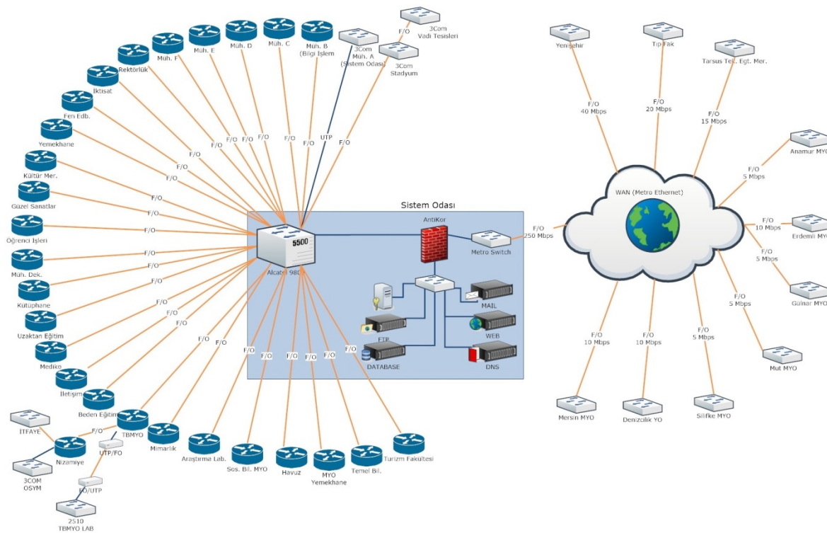
Şekil 3. Mersin Üniversitesi Bilgi İşlem Ağ Topolojisi
