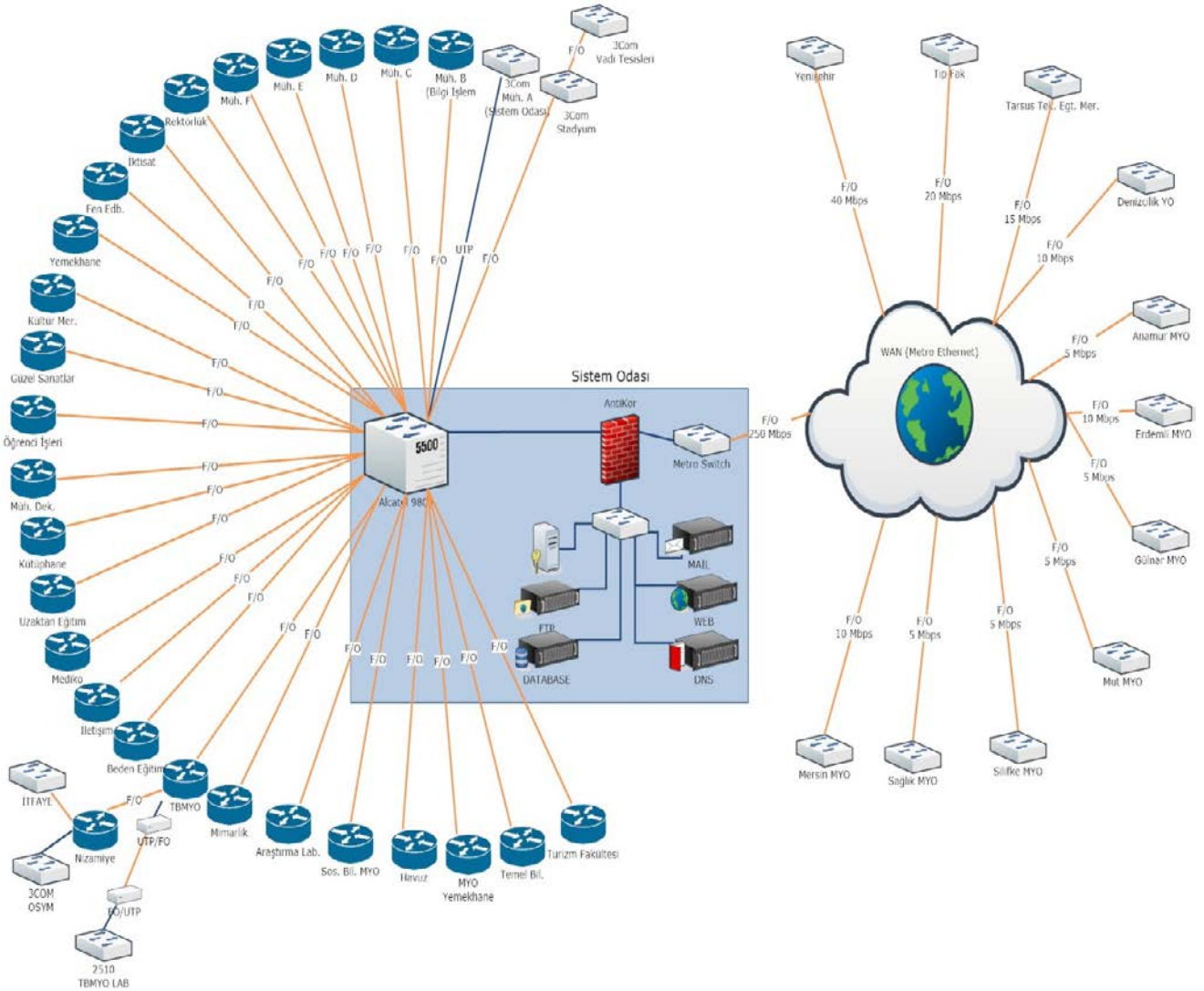
Şekil 3. Mersin Üniversitesi Bilgi İşlem Ağ Topolojisi
