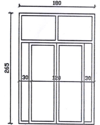
180/265 ALUMINYUM FOTOSELLİ KAPI
