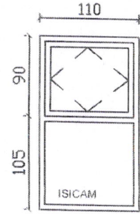
D7 GÖRÜNÜŞ
