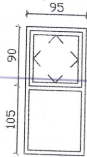
D4 GÖRÜNÜŞ
