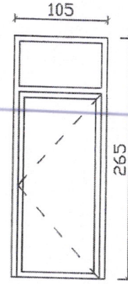
D12 GÖRÜNÜŞ
