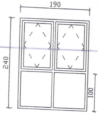
D1,D2,D6 (3 ADET)
