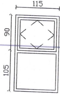
D3 GÖRÜNÜŞ
